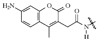
Coumarin
