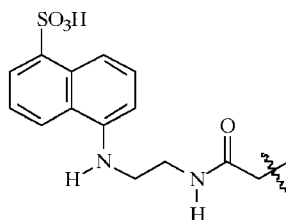
EDANS
