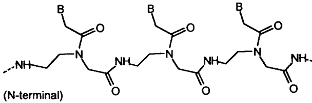
PNA
