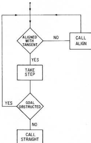
Fig. 6. Subalgorithm HUG.
