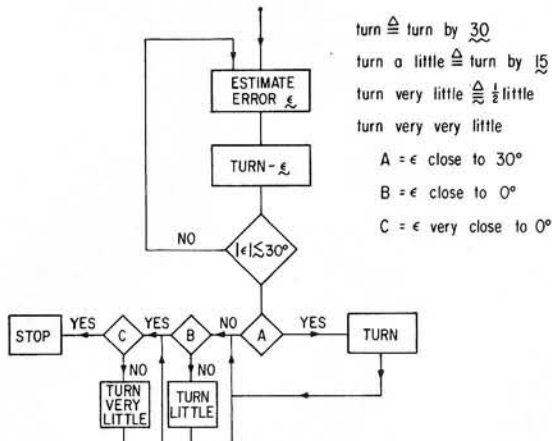
Fig. 5. Subalgorithm ALIGN.
