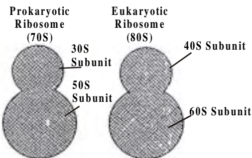
Fig : 2.18. Ribosome
