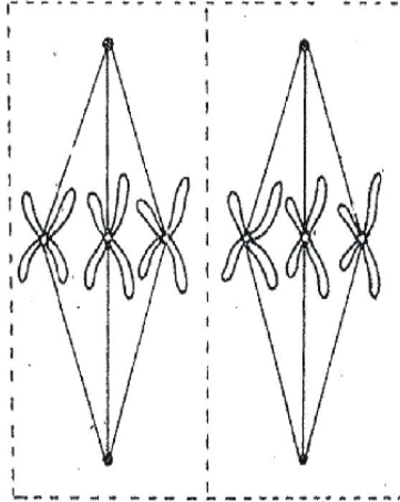
Telophase-II
