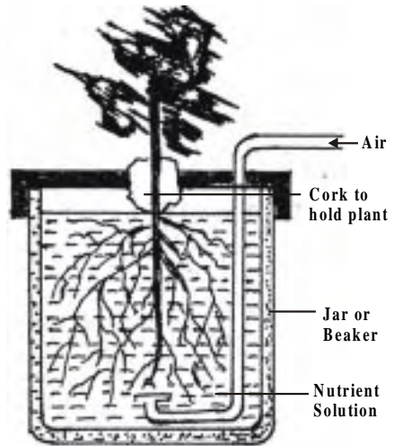
Fig : 5.7. Hydroponics
