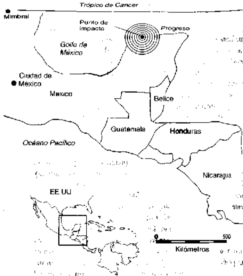
El vasto cráter de la península del Yucatán, formado hace unos 65 millones de años, es la prueba del deje de la extinción del Cretácico: el impacto de un asteroide.
