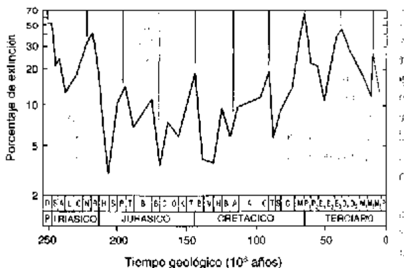
Según ciertas opiniones, las grandes extinciones se producen cada 26 millones de años, de manera periódica, las Cinco Grandes también. Se ha sugerido como causa el bombardeo periódico de asteroides que sufre la Tierra. (Reproducido por gentileza de David Raup y Jack Sepkoski.)
