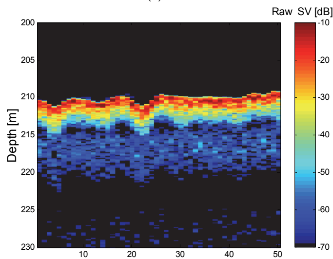
(b) Silt
